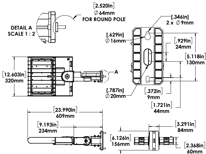
MONTAGE SUR RACCORD LISSE AVEC ADAPTATEUR
