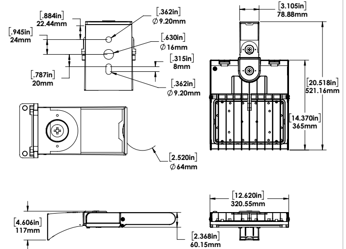
MONTAGE SUR BRAS
