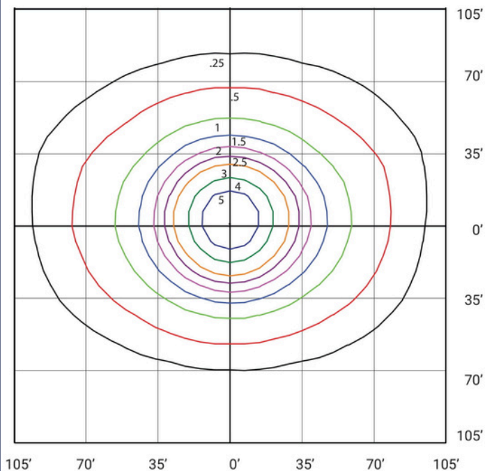
HELIX2-LED240A180-H-VK-T4-DIM-SP10 (240W, 120V, 4000K) INSTALLÉ À 10.7 MÈTRES (35 PIEDS)
