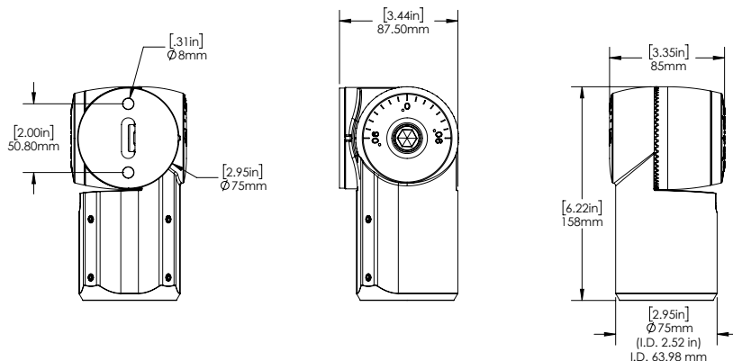
Montage à raccord lisse pour tourillon de 2 3/8 po Installation en usine optionnelle
