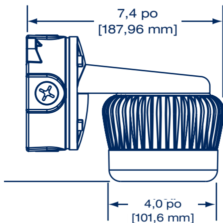
DVBKS-LED Au mur
