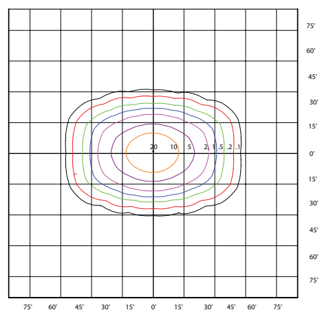
FL8A-LED300 ALLONGÉ TYPE V / 7H X 6V
