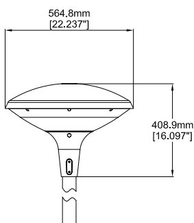
FL - Dessus plat
