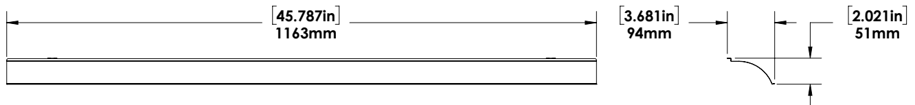
Wings dimensions
